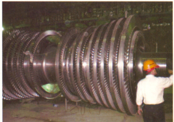
圖2. 1號機高壓汽機轉子維護保養作業
